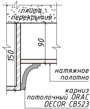
Разрез 2-2. М 1:5
