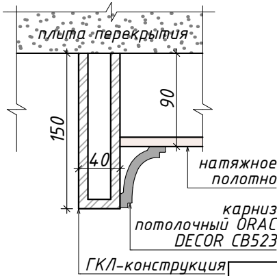
Разрез 1-1. М 1:5
